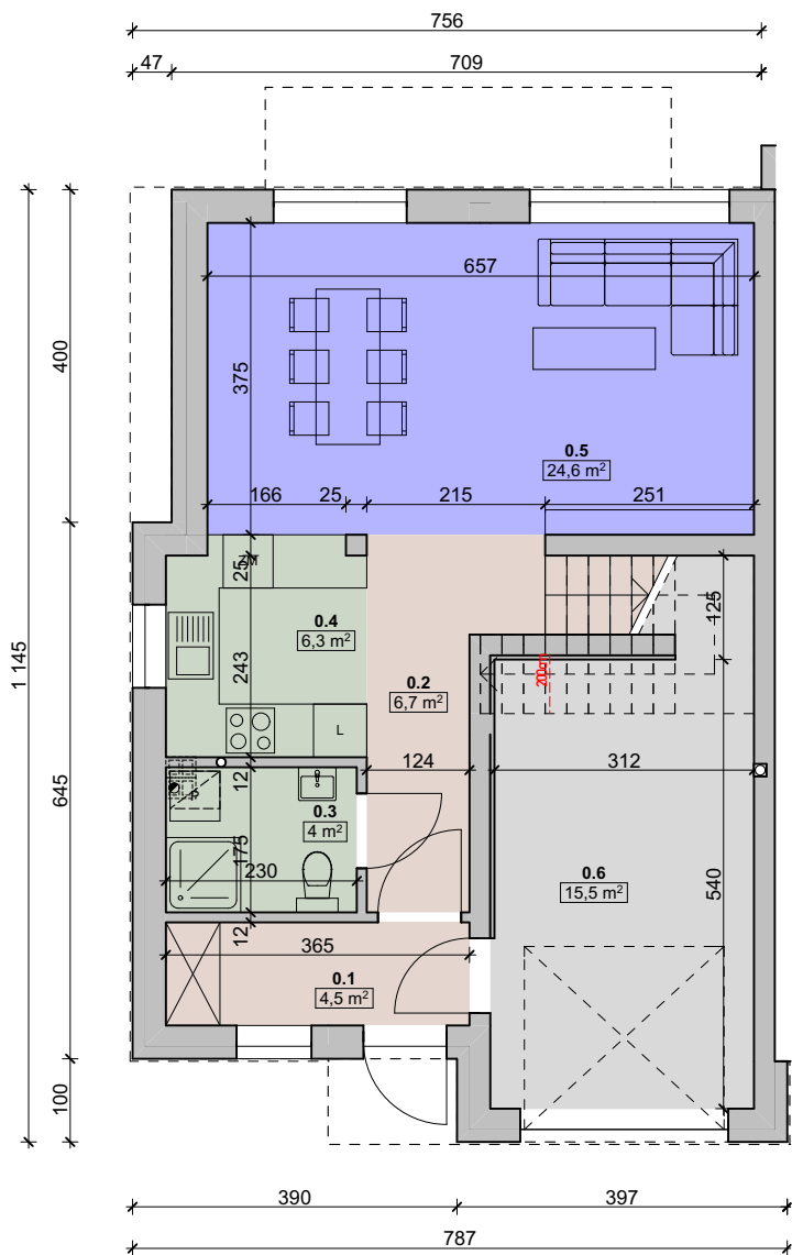
rzut parteru
