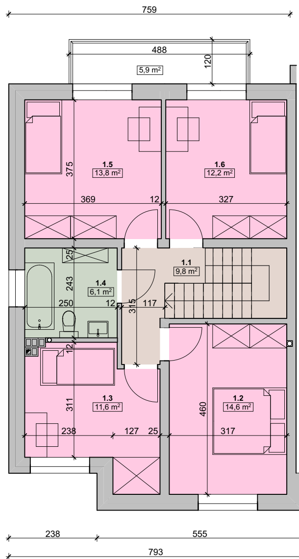
rzut piętra
