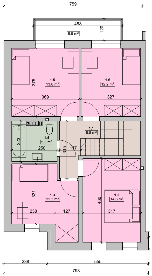
rzut piętra
