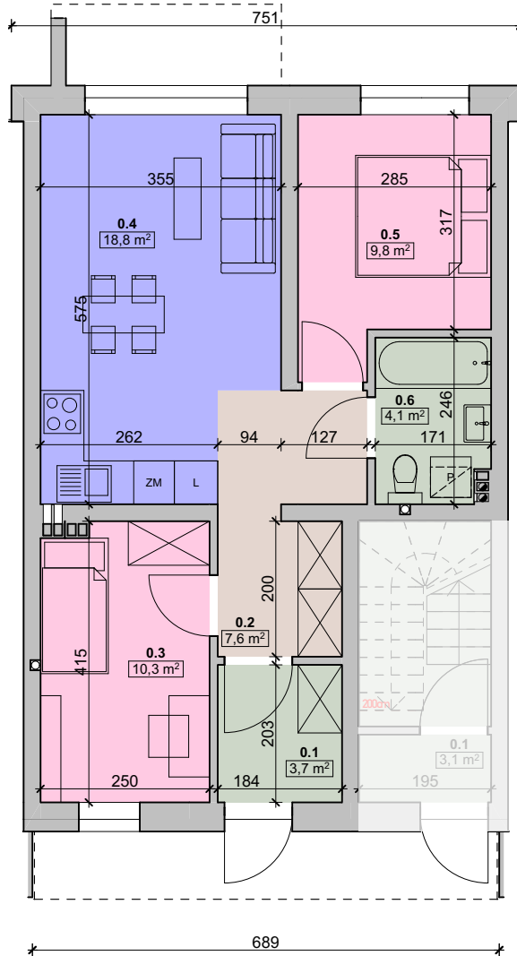
rzut parteru
